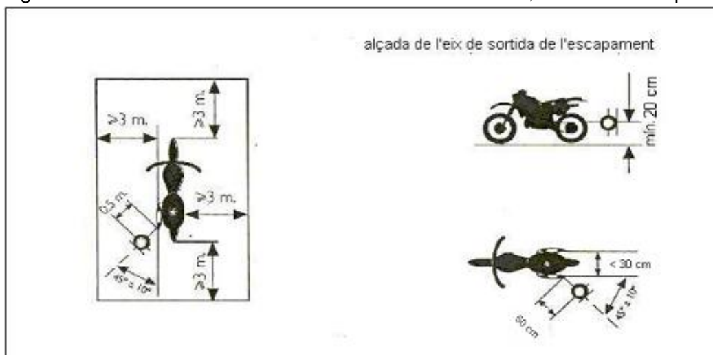
Figura 1. Posició de l'instrument de mesura en ciclomotors, motocicletes i quadricicles.
