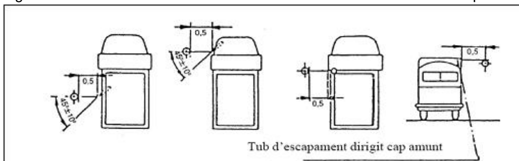
Figura 2. Posició de l'instrument de mesura en vehicles amb tub d'escapament vertical.
